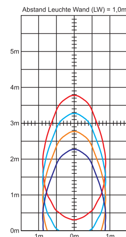
Lampenlichtstrom Not (DC) / Netz: 190lm / 190lm
