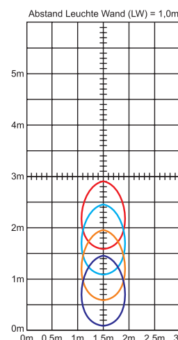
Mit min. 5lx angestrahlte Fläche bei Leuchtenhöhe(Lh) Lh=4,0m — Lh=3,5m — Lh=3,0m — Lh=2,5m —
