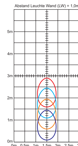
Lampenlichtstrom Not (DC) / Netz: 80lm / 190lm
