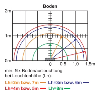
Lampenlichtstrom Not (DC) / Netz: 190lm / 190lm
