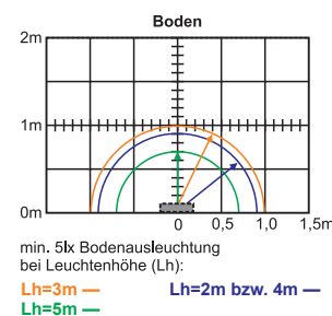
Lampenlichtstrom Not (DC) / Netz: 80lm / 190lm
