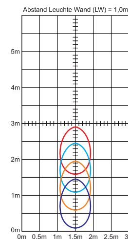
Mit min. 5lx angestrahlte Fläche bei Leuchtenhöhe(Lh)
