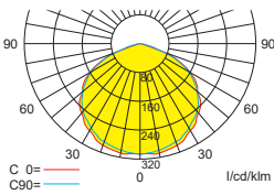
Leuchtmittel: 10W LED-Leiste Deckenmontage
